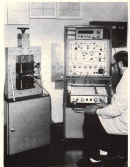
De hysteresislus van een magnetisch materiaal, kan men zien als zijn „identiteitsbewijs”. Met apparatuur van Krupp Forschungsinstitut kan men de hysteresislus d.m.v. een quasistatische meting bepalen, zonder dat het meetresultaat door drift onnauwkeuriger wordt.
