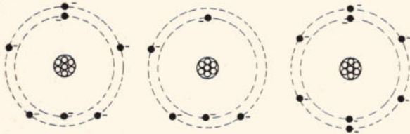
Fig. 19. Het aantal ladingen in de buitenste schil van een atoom kan worden gevarieerd:
