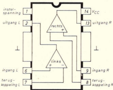
Fig. 1. Aansluitgegevens.
