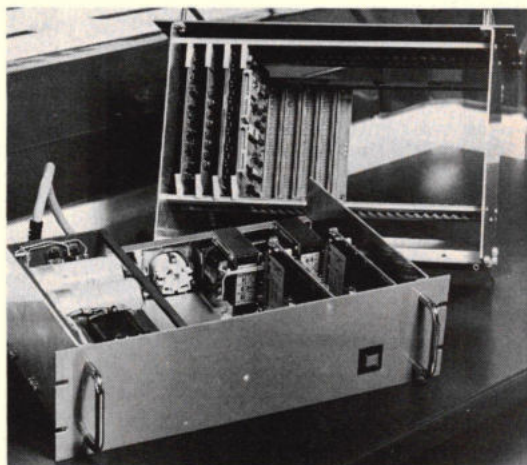
Afb. 18. Een microcomputer applicatie systeem.
