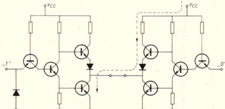
Fig. 1. Standaard TTL-poort, als „wired-OR” geschakeld.
