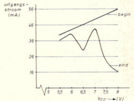
Fig. 3. Resultaten van de uitgangsstroom- en begrenzingstest. De basiswaarde werd gemeten toen de test werd ingeschakeld; de eindwaarde na twee uur in bedrijf.
