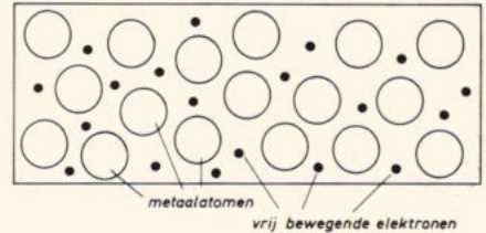
Fig. 20. Schematische atoomstructuur van een metaal. In de openingen tussen de atomen bevinden zich vrij bewegende elektronen.
